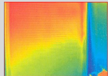
Thermografische Aufnahme an isolierverglastem Fenster mit Duette
